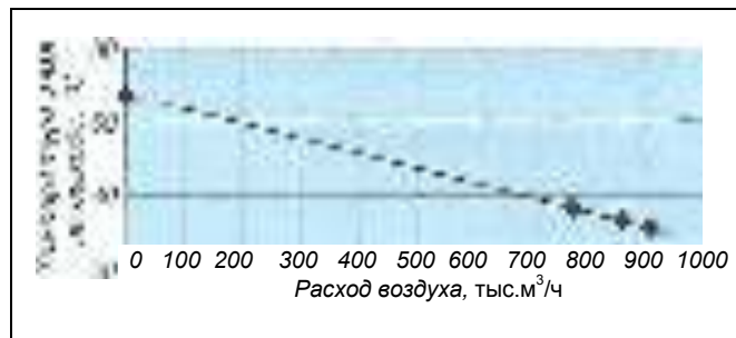
Рис. 2. Сравнение данных испытаний (♦) на КС «Курская» ООО «Мострансгаз» с результатом расчета (---) при расходе газа 357 тыс. м³/ч и температуре воздуха на входе 13°C
